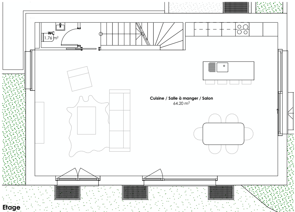
Etage 1/100°
