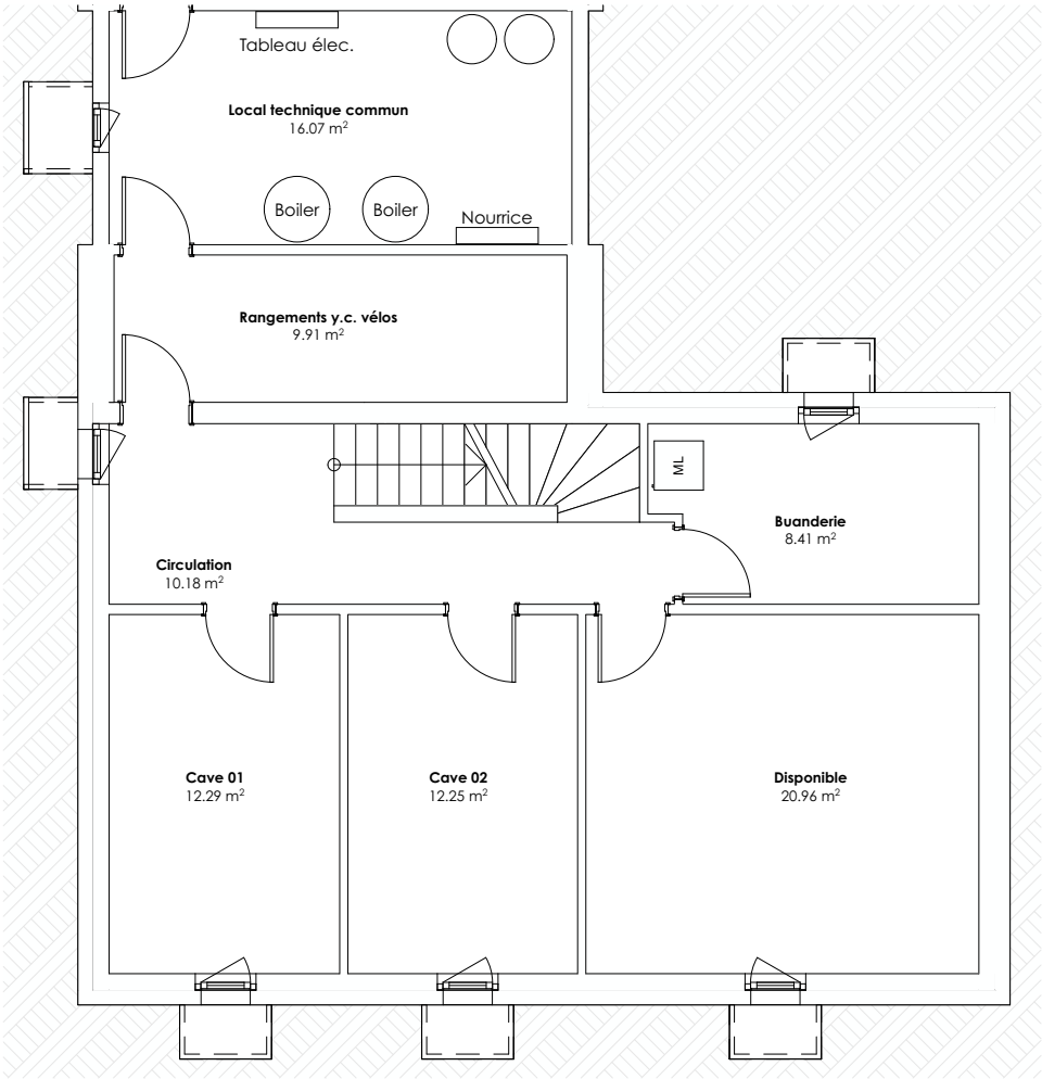
Sous-sol 1/100°
