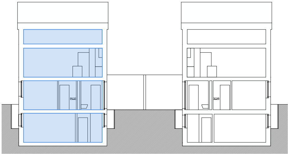
Coupe AA 1/200°
