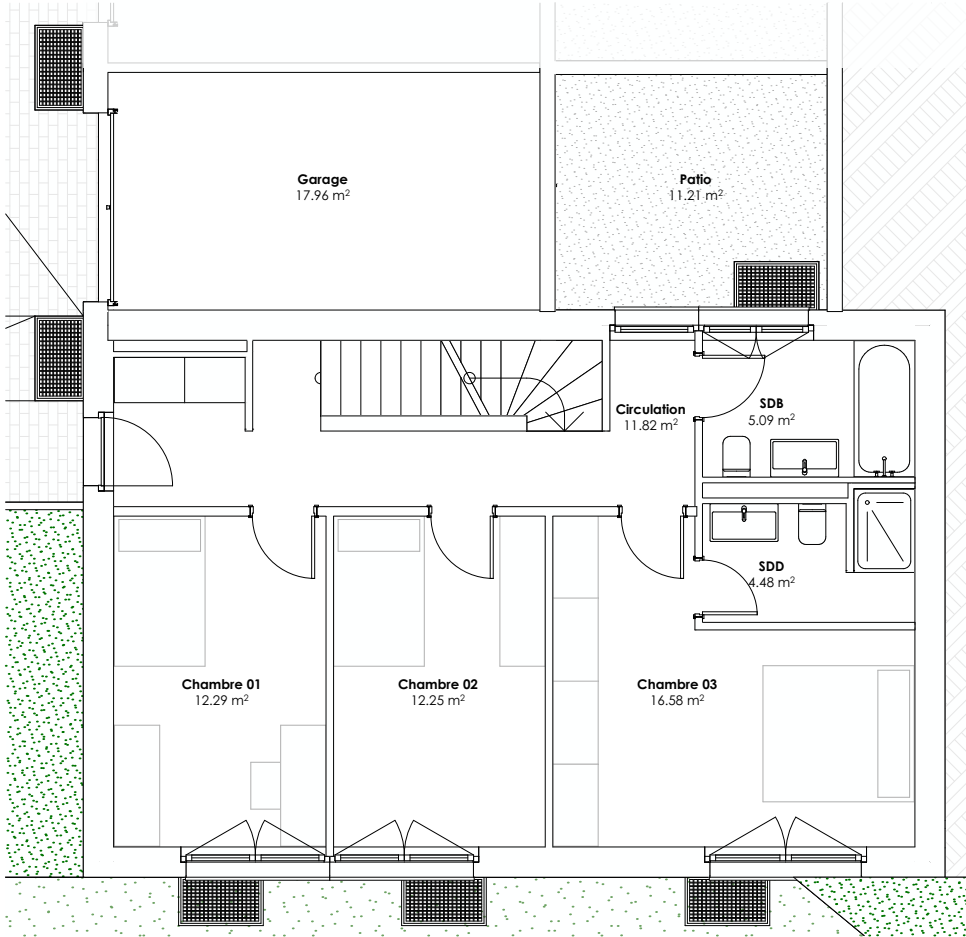
Rez-de-chaussée 1/100°
