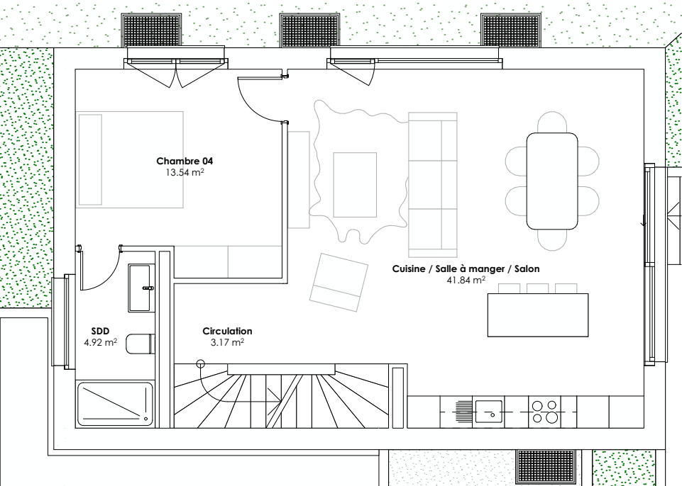
Étage 1/100 e
