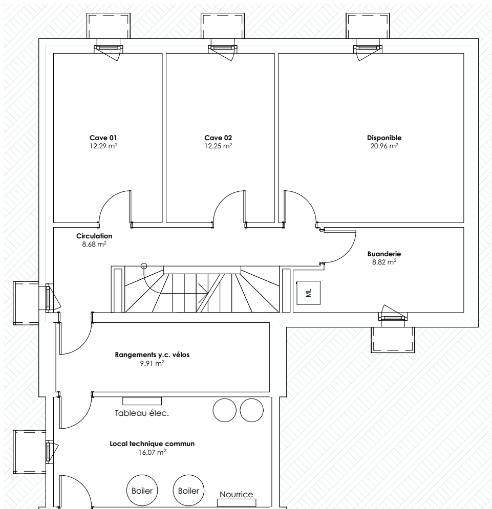
Sous-sol 1/100 e
