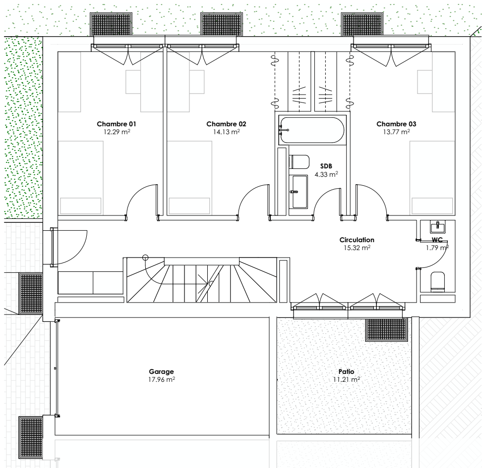
Rez-de-chaussée 1/100 e
